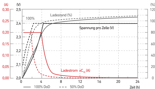
Ladung mit konstanter Spannung 2,40 V pro Zelle bei 20 °C und begrenztem Strom 0,2 C 10 A
